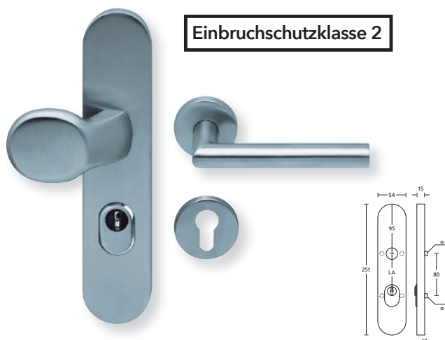
Schild/Rosettenkombination Einbruchschutzklasse 2 nach DIN EN 1906 mit Griffknopf
